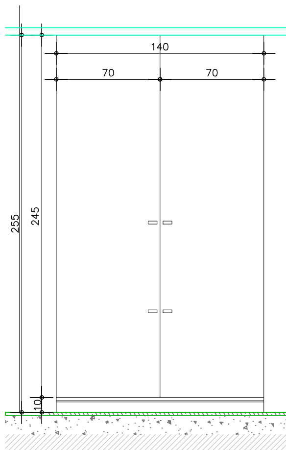
חזית
