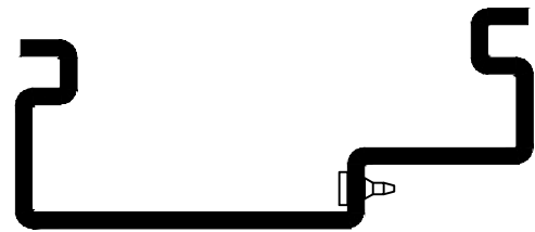
פרט משקוף 1:5
